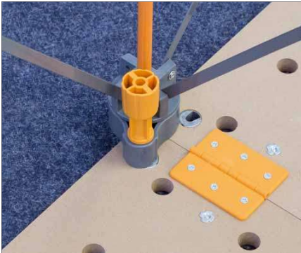
Um die Tischplatte zu fixieren werden die Haltebolzen von unten durch die Aufnahme am Untergestell in die Tischplatte gesteckt und durch verdrehen gesichert
