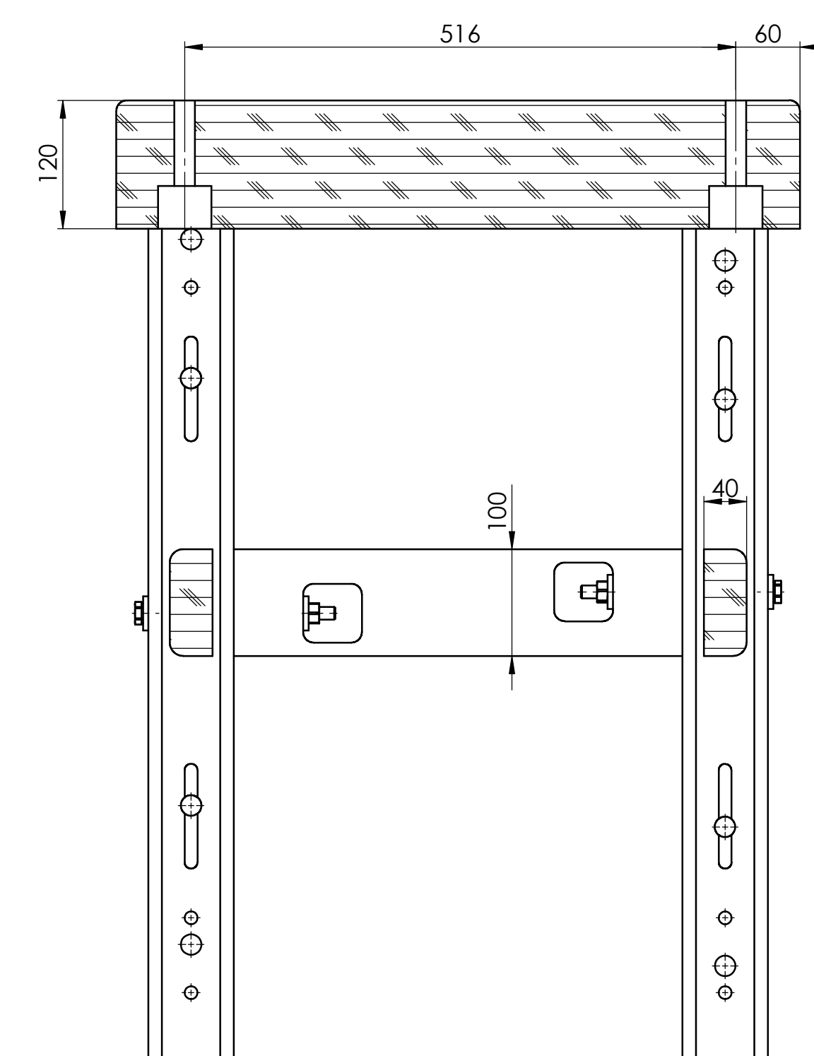
ŘEZ A-A MĚŘITKO 1 : 5
