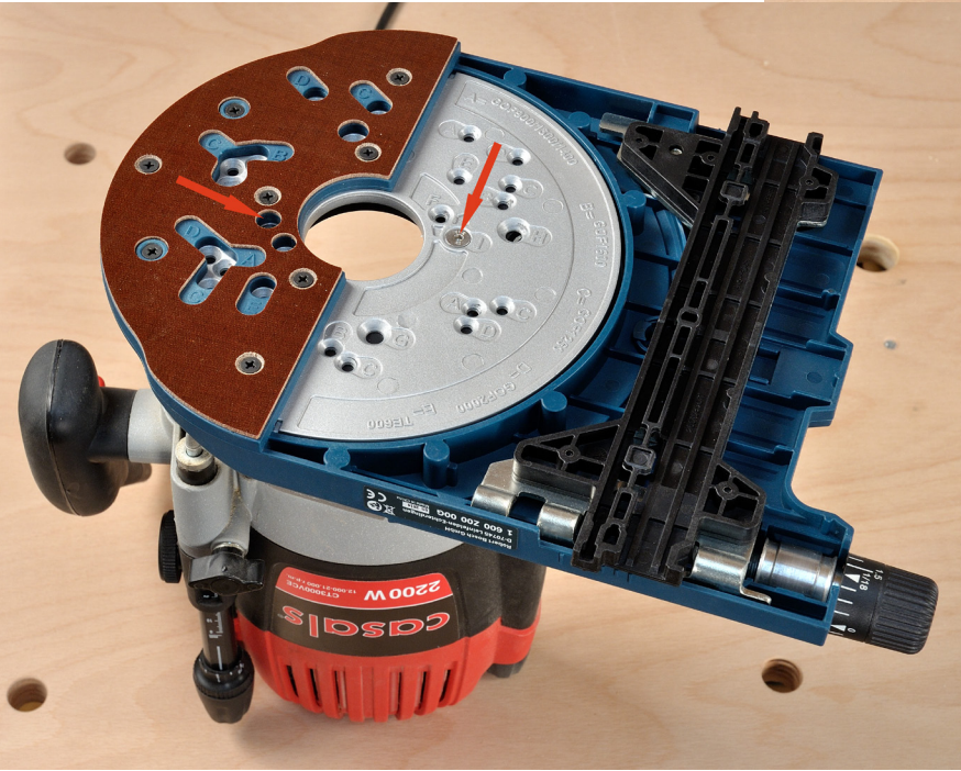
Die beiden mit „I“ bezeichneten Löcher im Adapter (Pfeile) sind die passenden Befestigungslöcher für die Casals/Freud Oberfräse.
