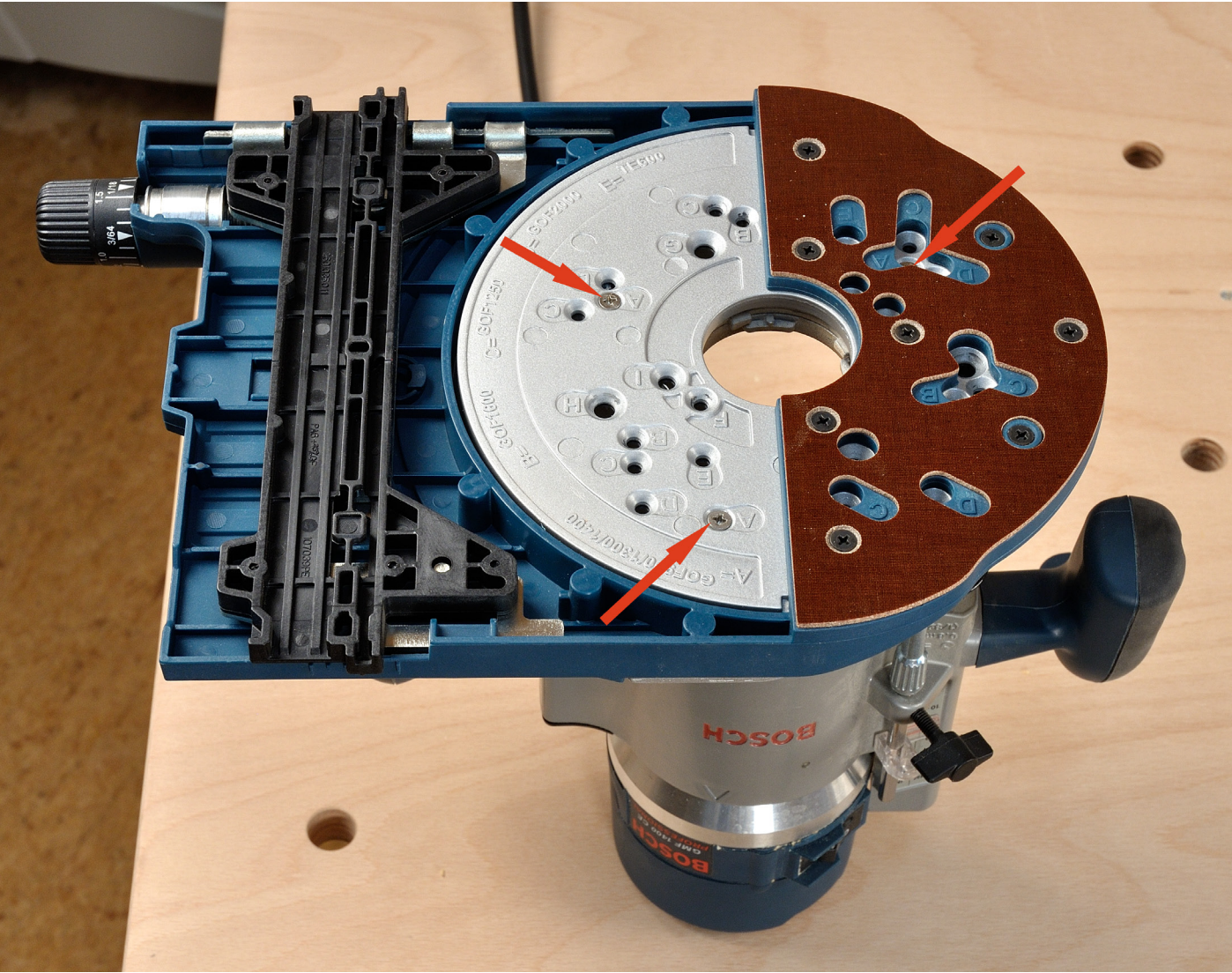
Auch ältere Bosch Oberfräsen wie z. B. die GMF 1400 (Bild) sind mit dem Adapter kompatibel. Weitere Bosch Modelle passen: GOF 900, 1250, 1300, 1400, 1600, 2000 und TE 600 (GKF 600).
