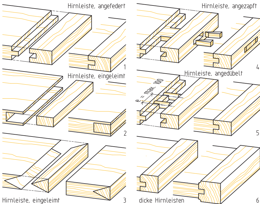
B 2.1-7 Hirnleisten, 1 angefedert und geleimt, 2 und 3 eingenutet und eingeleimt, 4 angezapft und sichtbar verkeilt, nur in der Mitte verleimt, 5 angedübelt und nur in der Mitte verleimt, 6 in der Dicke überstehende Hirnleistenformen.
