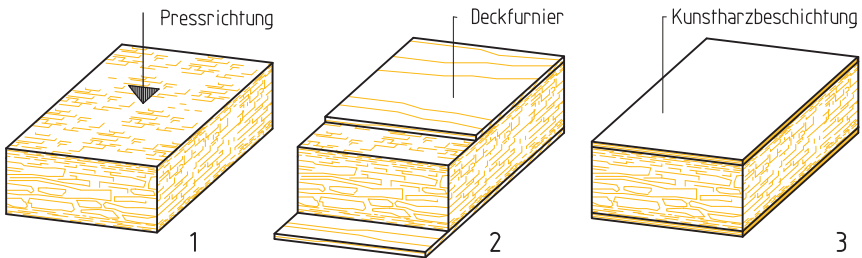
B 1.3-1 Spanplatten. 1 Flachpress-Spanplatte, mehrschichtig, 2 Flachpress-Spanplatte, furniert, 3 kunstharzbeschichtete (dekorative) Flachpressplatte.
