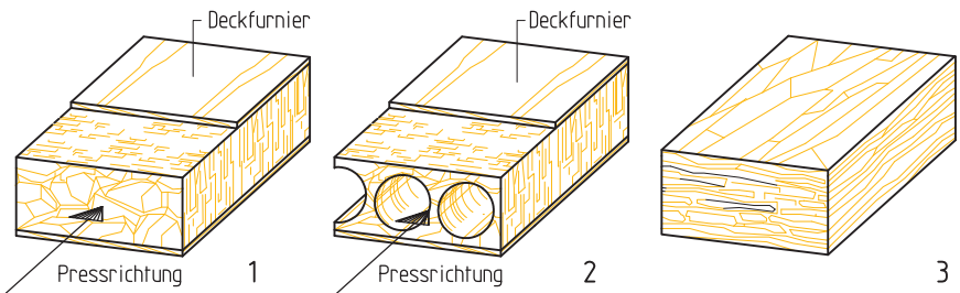
B 1.3-2 Besondere Spanplatten. 1 Strangpressplatte (ES), furniert, 2 Strangpress-Röhrenplatte (ET), 3 Langspanplatten (OSB-Platten).
