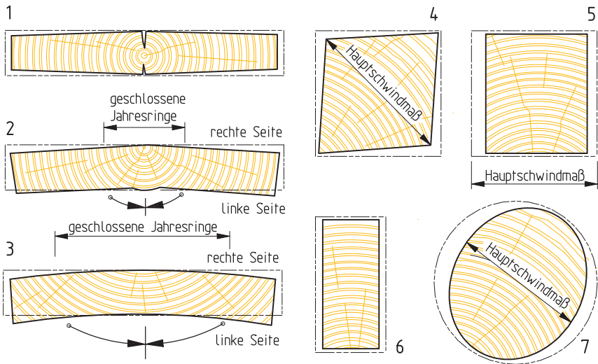
B 1.1-2 Die Schwindformen beim Schnittholz. 1 Herzblech mit nahezu mittlerer Markhöhle, 2 Mittelblech mit angeschnittener Markhöhle, 3 Seitenblech mit vielen nur einseitig angeschnittenen Jahresringen, 4 quadratisches Kantenholz mit vorwiegend diagonal laufenden Jahresringen und 5 mit kantenparallelen Jahresringen, 6 Brettstück mit stehenden Jahresringen und 7 Verformung eines kreisrunden Querschnitts.
