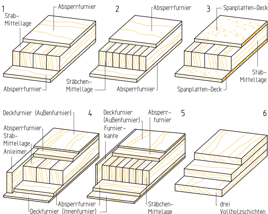
B 1.2-2 Verbundsperr Holz. 1 Stabsperr Holz, 2 Stäbchensper Holz, 3 Stabplatte mit Spanplatten decks, 4 Stabsperr Holz mit Anleimer und beidseitig überfurniert, 5 Stäbchensper Holz, beidseitig überfurniert, mit Furnierkante, 6 Dreischichtplatte.
