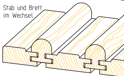
B 2.1-4 Die überschobene Schalung.
