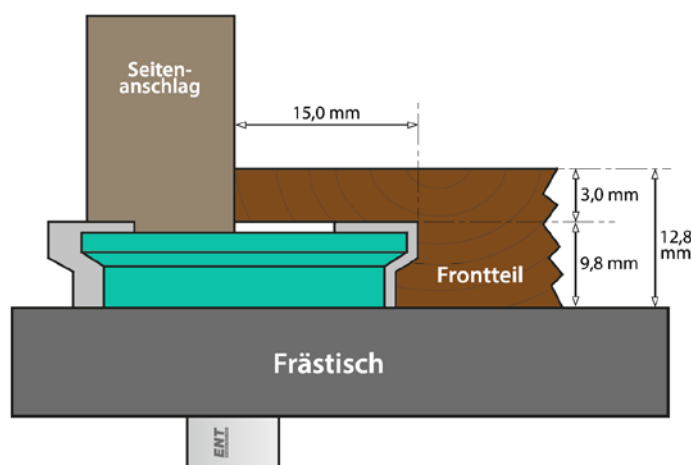
Abbildung 2: Frontteil fräsen
