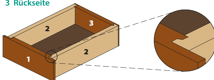
Abbildung 1: Frontteil mit seitlichem Überhang
