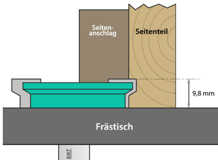
Abbildung 3: Seitenteil fräsen
