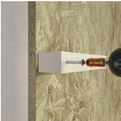
Befestigung einer Installationsebene
