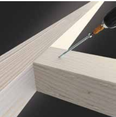
Haupt-Nebenträger-Verbindung
