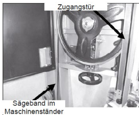
Sägeband im Maschinenständer
