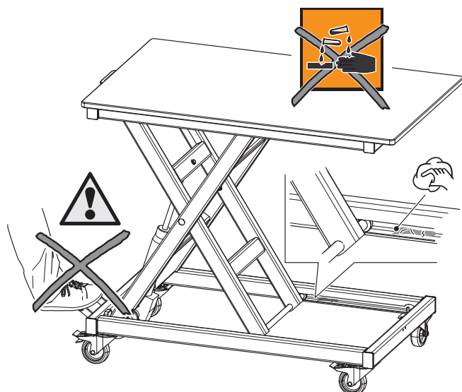
Abb. 7-1: Späne und Staub entfernen
