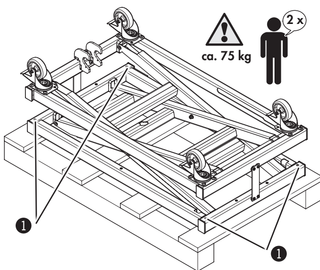
Abb. 4-1: Transportsicherung
