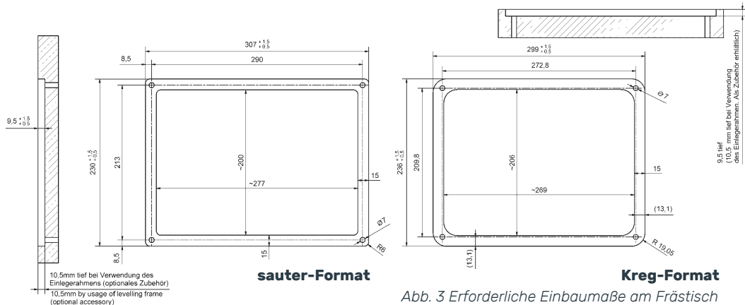
Abb. 3 Erforderliche Einbaumaße am Frästisch
