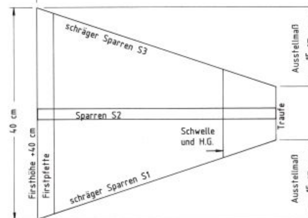
Grundriß / D1
