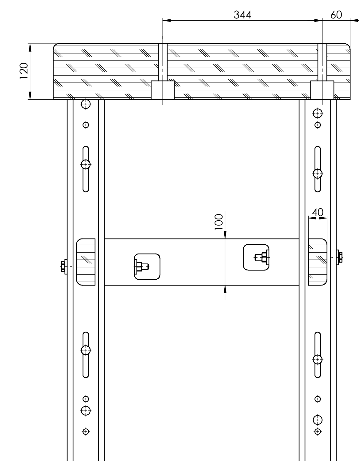
ŘEZ A-A MĚRITKO 1 : 5
